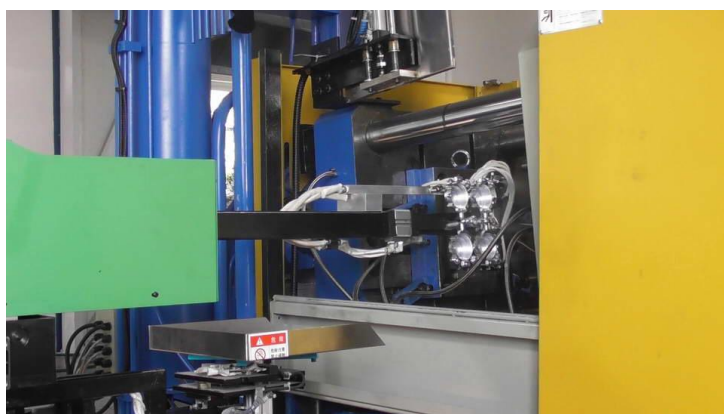
Машина для литья под давлением.
