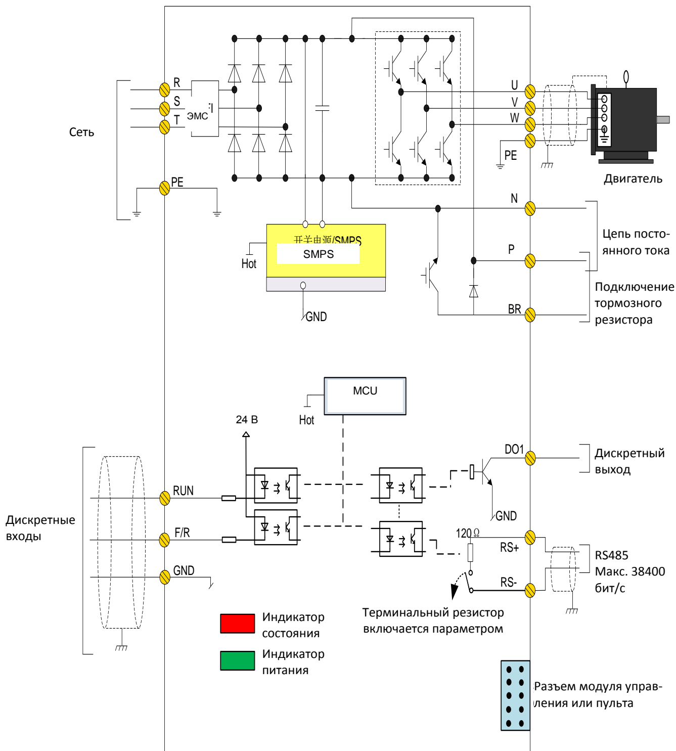
Силовой модуль PU01 (0.37-7.5 кВт)
