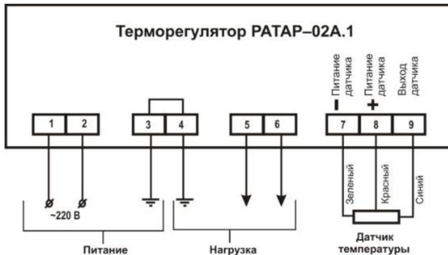
Схема электрическая подключения терморегулятора РАТАР-02.А1
