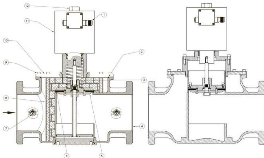
Конструкция версии 0,3-0,6 МПа
