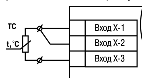
Рисунок 5.11 – Трехпроводная схема подключения ТС
