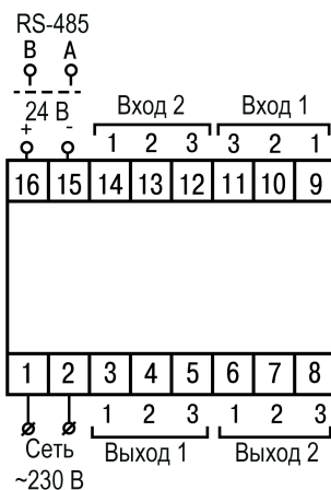
Рисунок 5.6 – Общая схема подключения ТРМ12–Д
