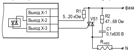
Рисунок 5.22 – Схема подключения силового симистора к ВУ типа «С»
