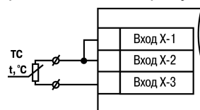
Рисунок 5.12 – Двухпроводная схема подключения ТС
