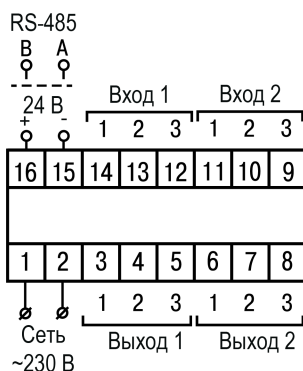
Рисунок 5.5 – Общая схема подключения ТРМ12–Ц5
