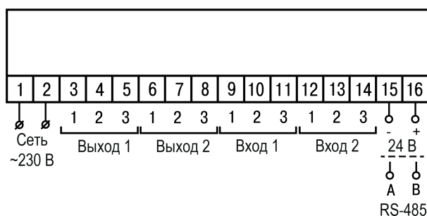
Рисунок 5.4 – Общая схема подключения ТРМ12–Щ1/Щ2
