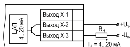
Рисунок 5.24 – Подключение к ВУ типа «И»
