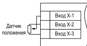
Рисунок 5.18 – Подключение датчика положения резистивного типа
