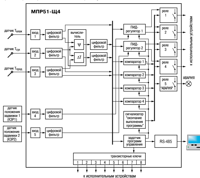
Рисунок 6.1 – Функциональная схема прибора
