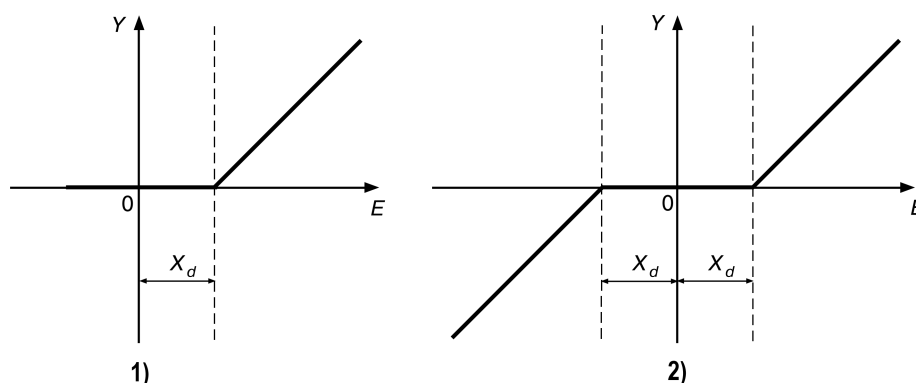
Рисунок 7.17 – 1) Зона нечувствительности для исполнительного устройства типа «нагреватель» 2) Зона нечувствительности для исполнительного устройства типа «нагреватель — холодильник» или «задвижка»
