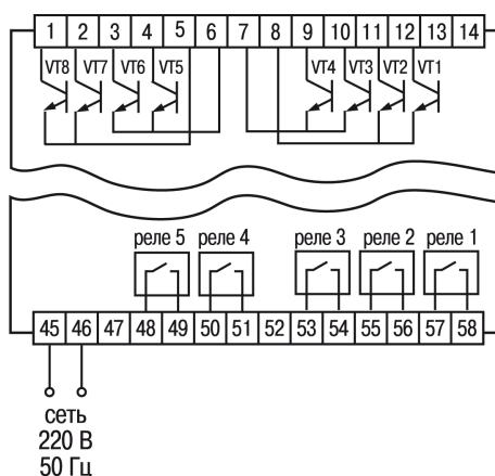
Рисунок 5.4 – Подключение измерительных датчиков и датчиков положения задвижек
