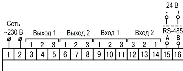
Рисунок 5.7 – Общая схема подключения 2TRM1–Н
