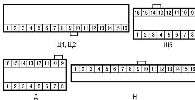
Рисунок 7.9 – Установка перемычки
