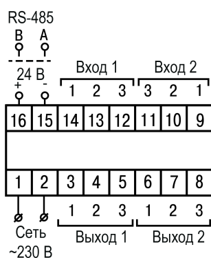
Рисунок 5.5 – Общая схема подключения 2TRM1–Ц5
