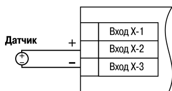
Рисунок 5.13 – Схема подключения активного датчика с выходом в виде напряжения -50\dots+50 мВ или 0\dots1 В
