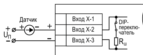
Рисунок 5.14 – Схема подключения пассивного датчика с токовым выходом 0\dots5 мА или 0 (4) \dots20 мА
