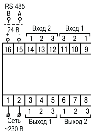
Рисунок 5.6 – Общая схема подключения 2TRM1–Д
