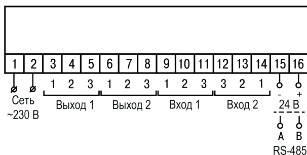
Рисунок 5.4 – Общая схема подключения 2ТРМ1–Щ1/Щ2
