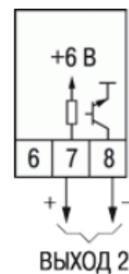
ВУ2 типа Т (для управления твердотельным реле)
