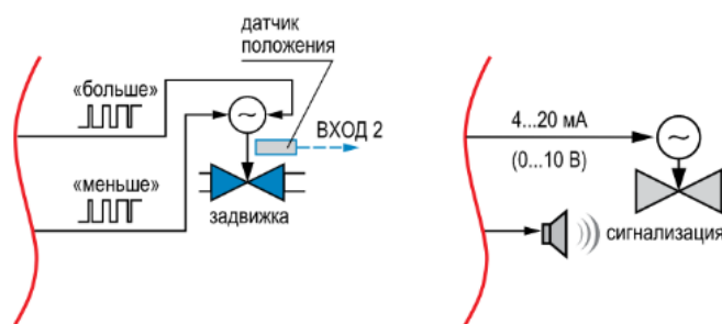
ПИД-регулирование с помощью задвижки с аналоговым управлением
