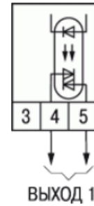
ВУ1 типа С (симисторная оптопара)
