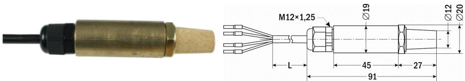
Рис. 4 – Датчик температуры и влажности ARHT-13C
