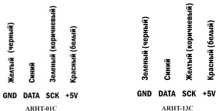
Рис. 6 – Схемы подключения датчиков.
