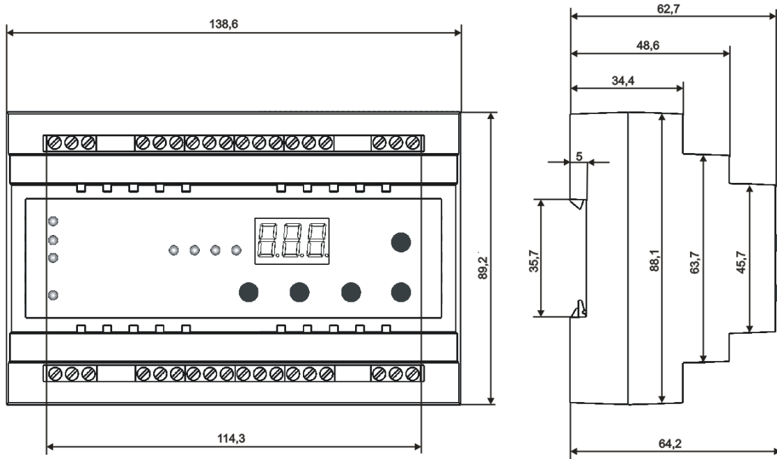
Рисунок 3.1 – Габаритные размеры прибора
