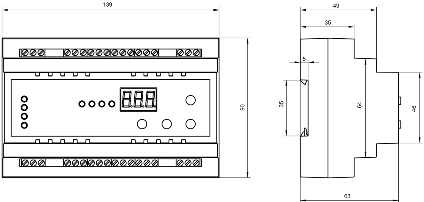
Рисунок 3.1 - Габаритные размеры прибора
