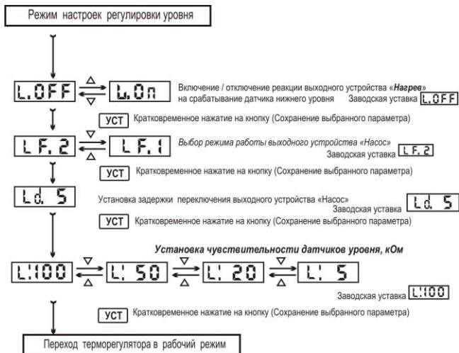
Рисунок 5 – Алгоритм программирования терморегулятора PATAP-02U (продолжение)
