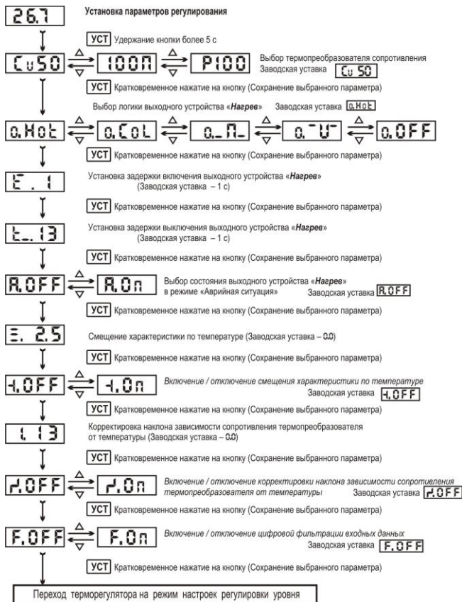
Рисунок 5 – Алгоритм программирования терморегулятора РАТАР-02У (см. продолжение на следующей странице)
