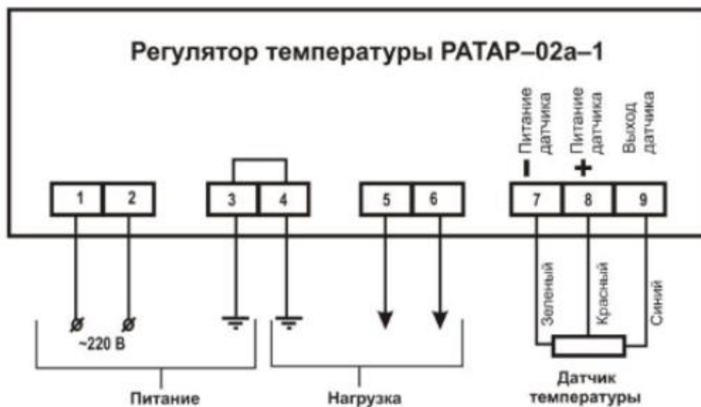
Схема электрическая подключения регулятора температуры RATAR-02a-1
