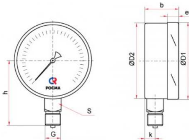
Радиальное присоединение
