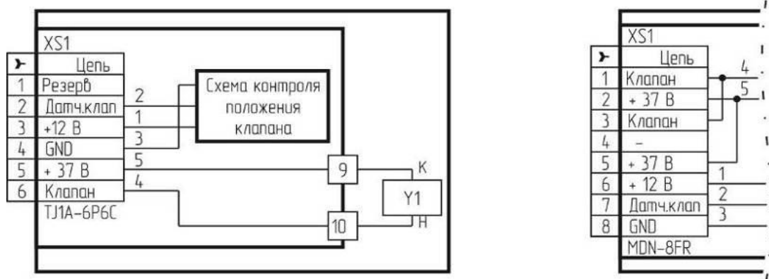
а) с разъемом типа TJ1A-6P6C
