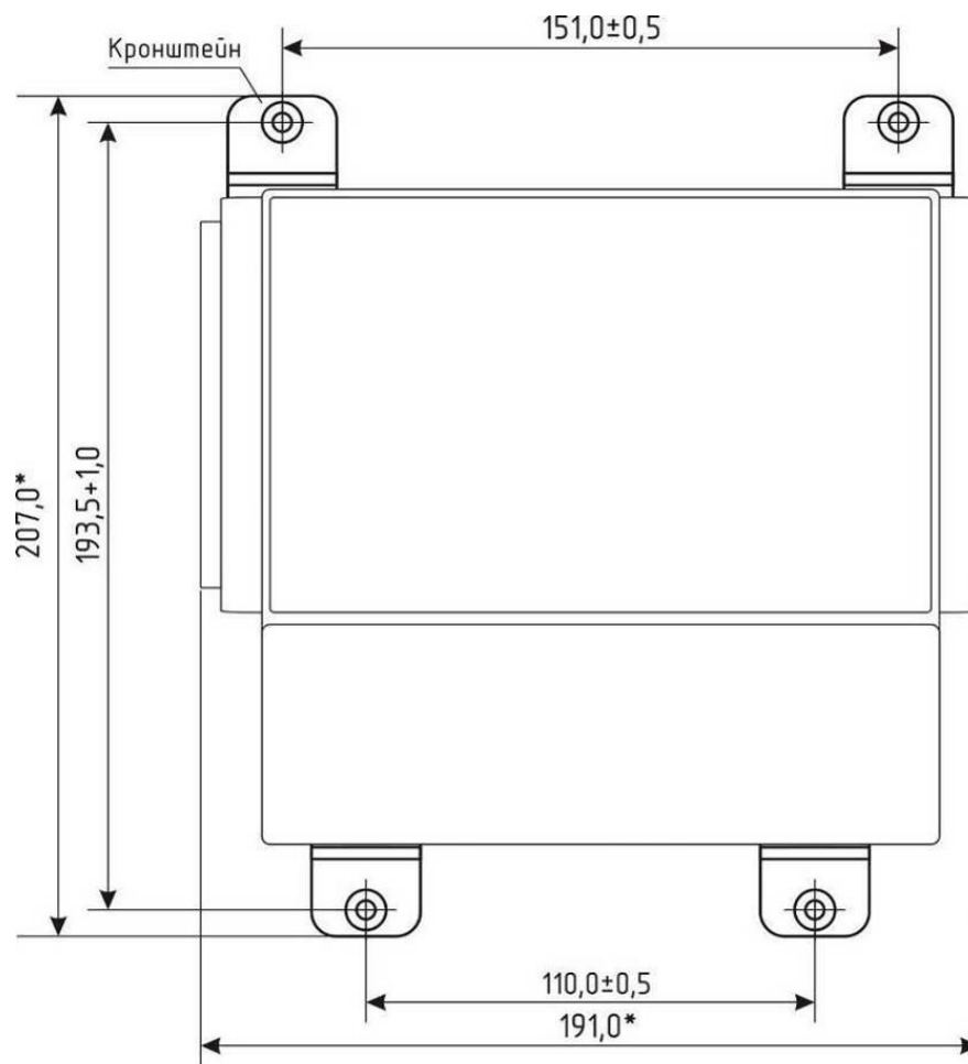
Рисунок Г.1 – Разметка отверстий для крепления сигнализаторов СЗ-1Е (-2Е, -3Е), пульта
