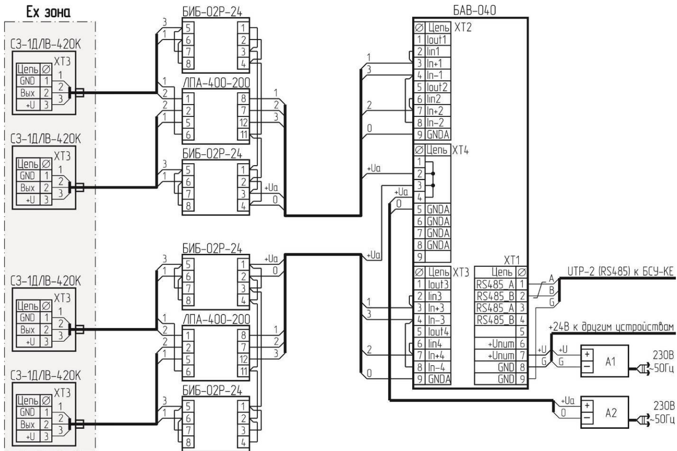
Рисунок А.2 – Схема подключения барьеров искрозащиты.
