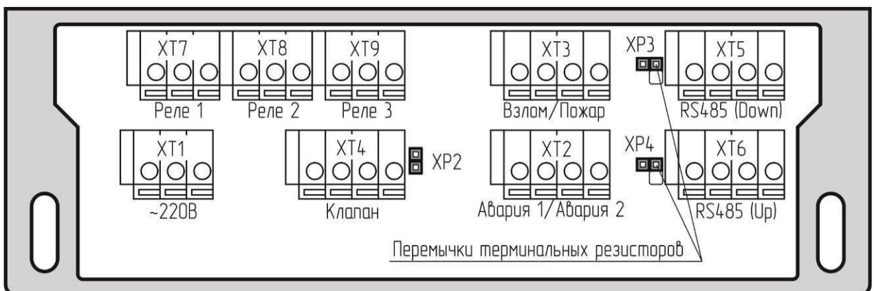
Рисунок Г.7 – Расположение клеммников БСУ-КЕ
