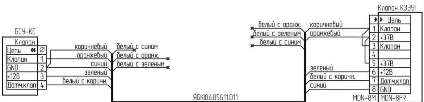
Рисунок А.6 – Типовая схема подключения клапана КЗЭУГ с разъемом MDN-8FR
