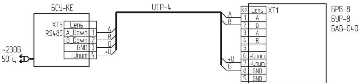
Рисунок 13 – Схемы соединений для программирования адресов
