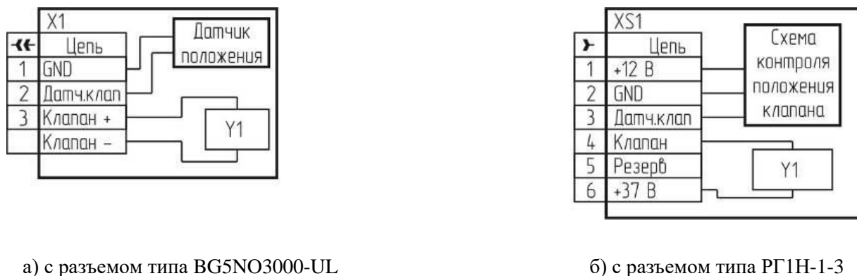
Рисунок 6 – Клапан КЗГЭМ-У. Схема электрическая принципиальная.
