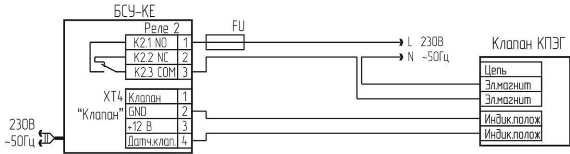
а) схема подключения клапана типа КПЭГ
