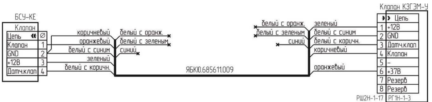
Рисунок А.4 – Типовая схема подключения клапана КЗГЭМ-У с разъемом PG1H-1-3
