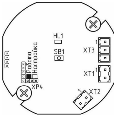
Рисунок Г.8 – Схема расположения разъемов СЗ-1ДЛВ-420К
