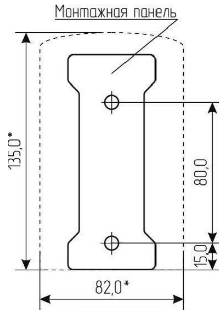
Рисунок Г.1 – Разметка отверстий для крепления сигнализаторов СЗ-1Е (-2Е, -3Е), пульта
