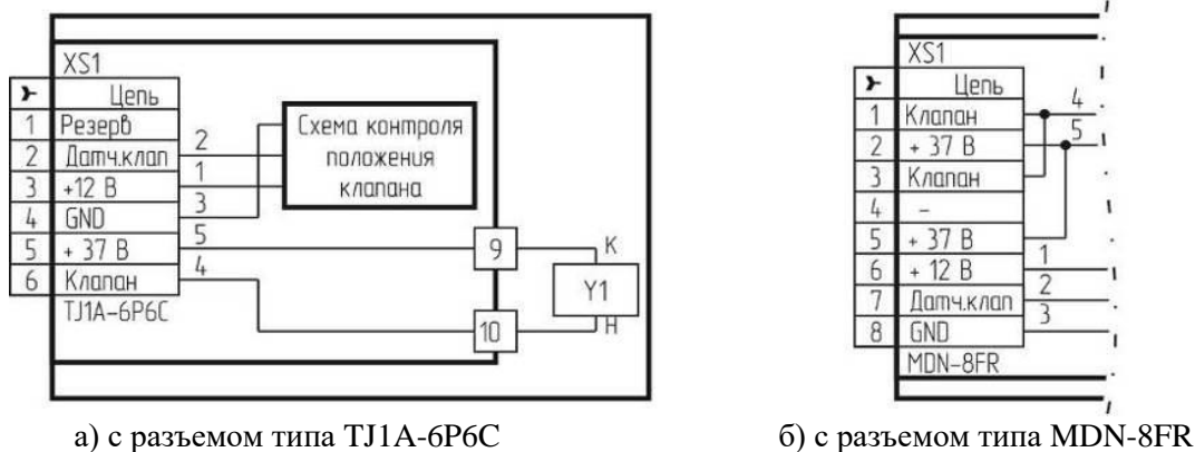
Рисунок 4 – Клапан КЗЭУГ. Схема электрическая принципиальная.
