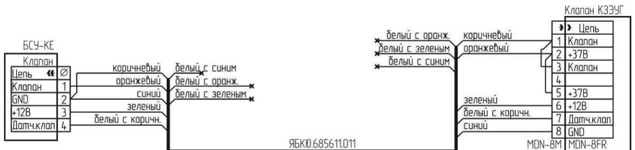
Рисунок Г.6 – Типовая схема подключения клапана К3ЭУГ с разъемом MDN-8FR
