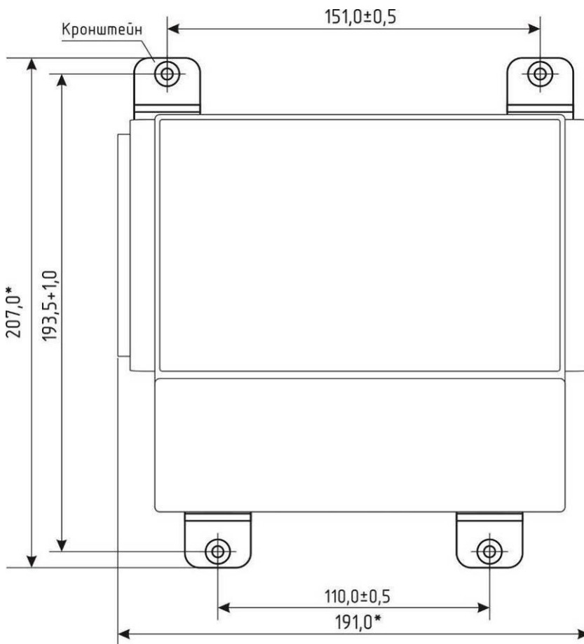
*Размер для справок Рисунок В.2 – Разметка отверстий для крепления БСУ-КЕ
