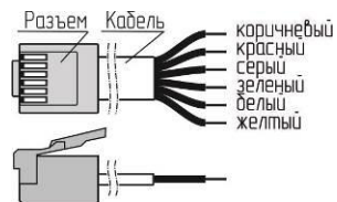
Вилка на кабель TR6P6C (цвета проводов)
