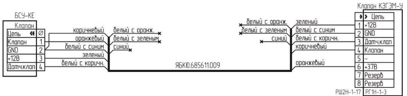
Рисунок Г.4 – Типовая схема подключения клапана К3ГЭМ-У с разъемом PG1H-1-3
