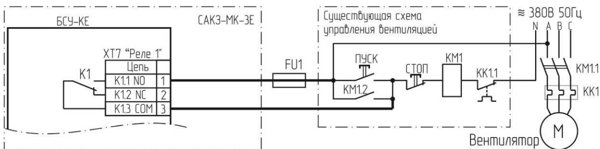
Рисунок Г.9 – Типовая схема соединений для управления вентиляцией
