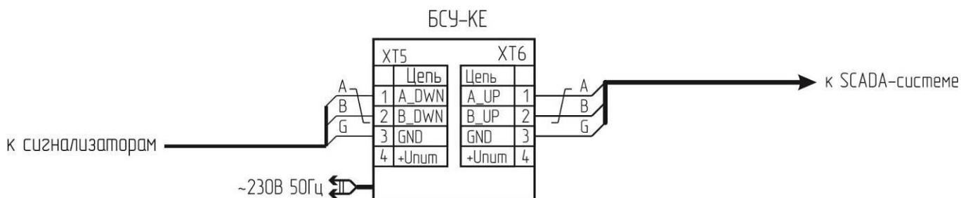
Рисунок 19 – Схема подключения к SCADA.
