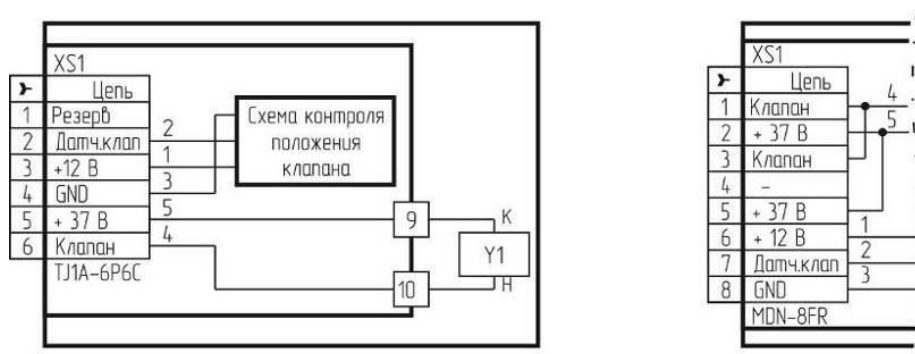
а) с разъемом типа TJ1A-6P6C
