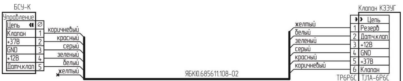
Рисунок Г.8 – Типовая схема подключения клапана КЗЭУГ с разъемом TJ1A-6P6C
