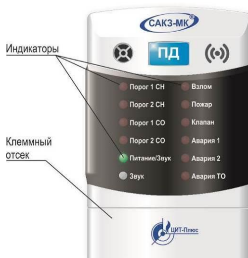
Рисунок 9 – Внешний вид пульта
