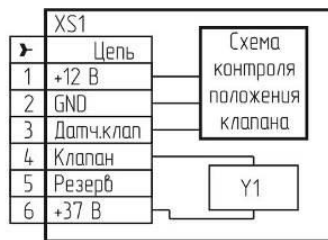
б) с разъемом типа PГ1Н-1-3
