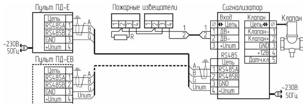
Рисунок 11 – Схема соединений системы с RS485, одним сигнализатором и пультом.
