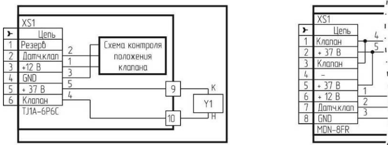
Рисунок 3 – Клапан КЗЭУГ. Схема электрическая принципиальная.
