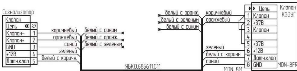
Рисунок В.3 – Схема подключения клапана КЗЗУГ с разъемом MDN8FR.
