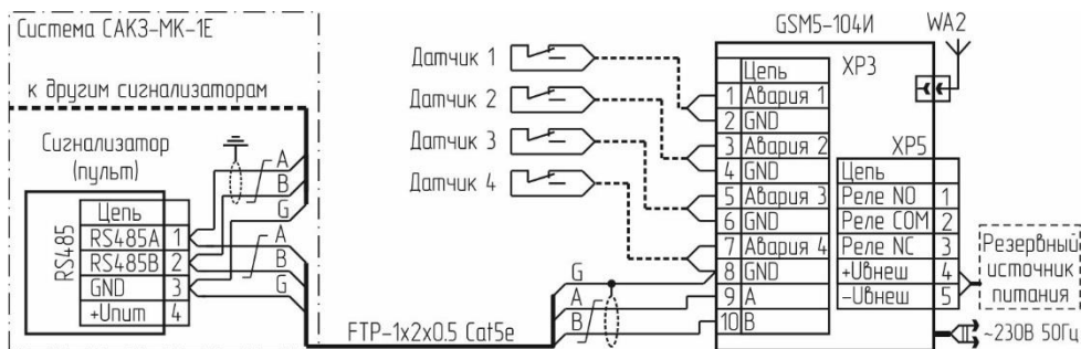
Рисунок В.6 – Схема подключения извещателя GSM5-104И.
