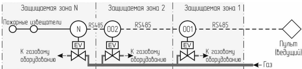
Рисунок 16 – Система с RS485 и индивидуальной защитой.
