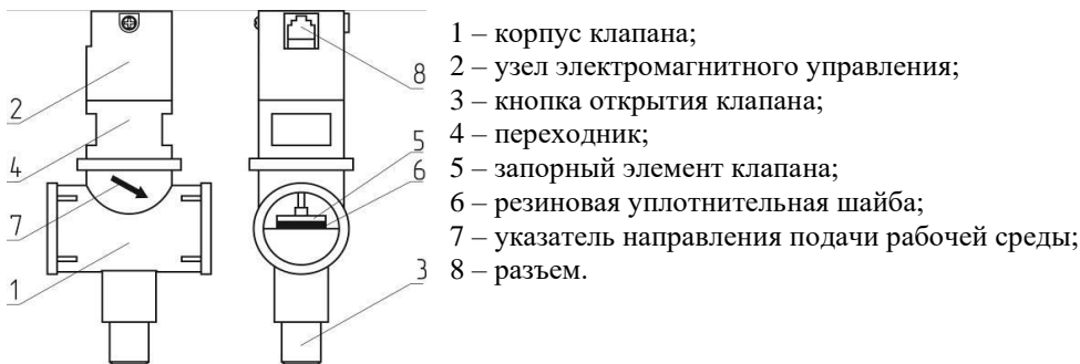
Рисунок 2 – Внешний вид клапана КЗЭУГ.
