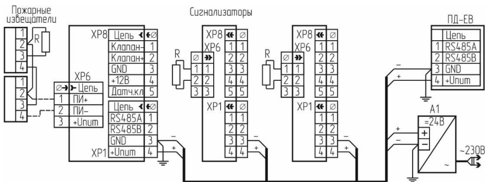
Рисунок В.6 – Схема подключения извещателя GSM5-104И.
