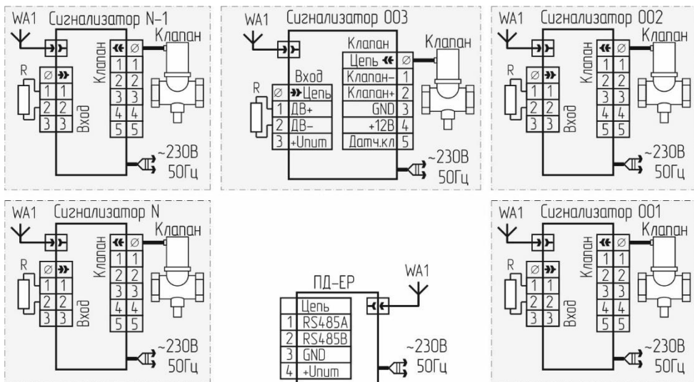
Рисунок 21 – Система с индивидуальной защитой и связью по радиоканалу
