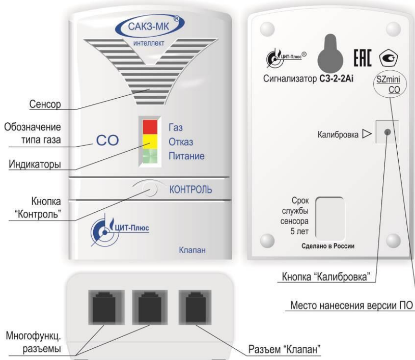
Рисунок 1 – Внешний вид сигнализатора.
