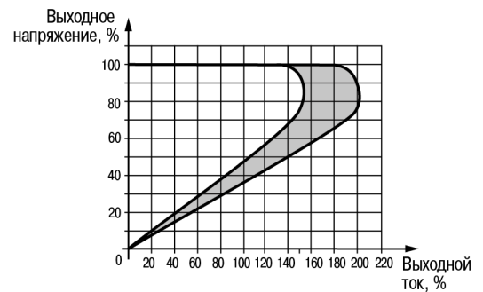
Рисунок 4 - График зависимости выходного напряжения от выходного тока
