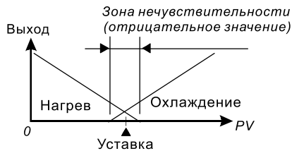
Рис 6: ПИД-регулирование. Двухконтурное управление с отрицательной зоной нечувствительности
