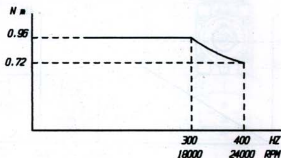
CURVE DELLA COPPIA Torque Curves
