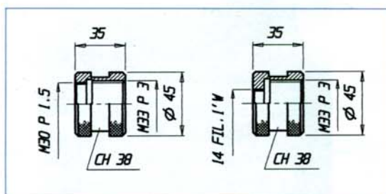
Ghiere per Cono Morse n° 2-3
