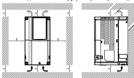
Рис. 1. Один ПЧ в шкафу (типоразмеры А-Н)
