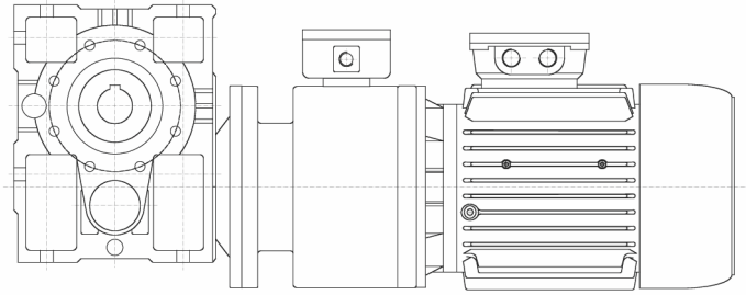
Стандартный двигатель B5 + тормоз VIS + редуктор
