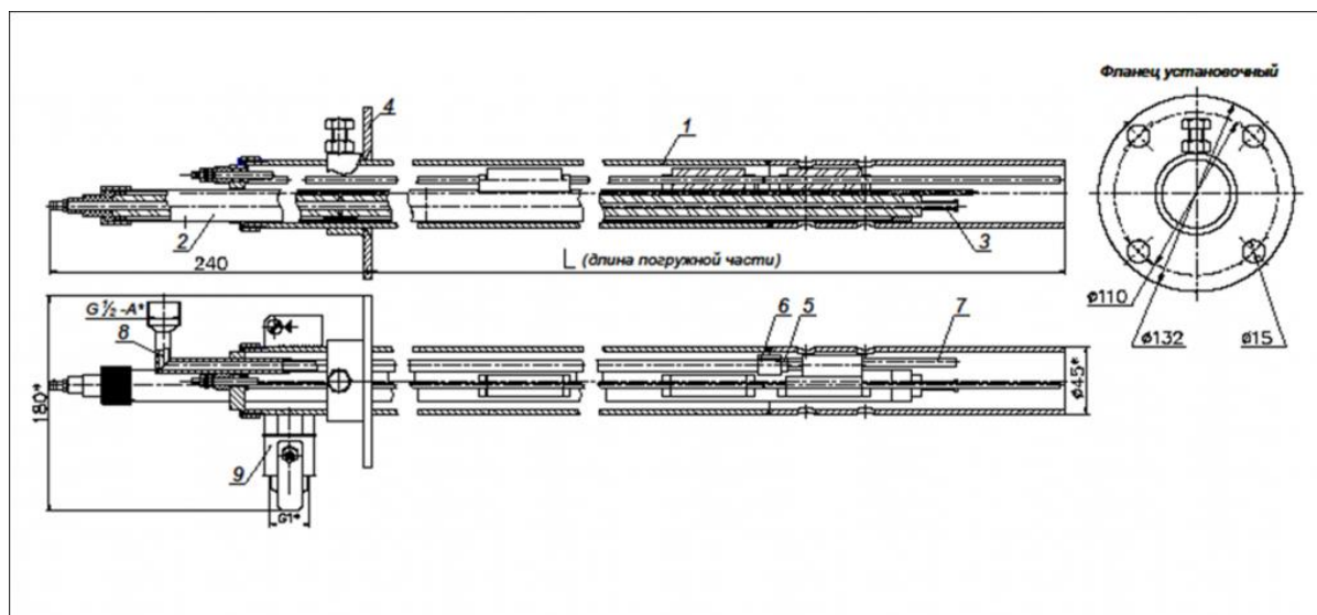
Общий вид запальной горелки инжекционной ЗГИ с диаметром ствола 45 мм.
