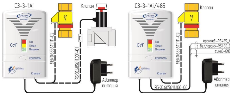
Рисунок Б.1 – Типовая схема включения сигнализатора
