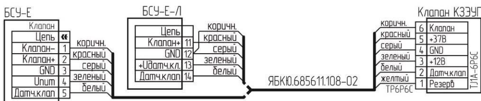
Рисунок Б.4 – Схема подключения клапана КЗЭУГ с разъемом T1A-6P6C
