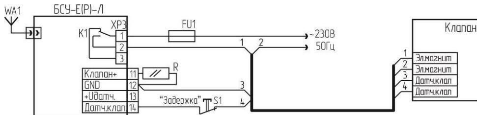
б) блок БСУ-Е(Р)-Л
