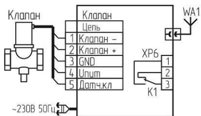
а) БСУ-ЕР
