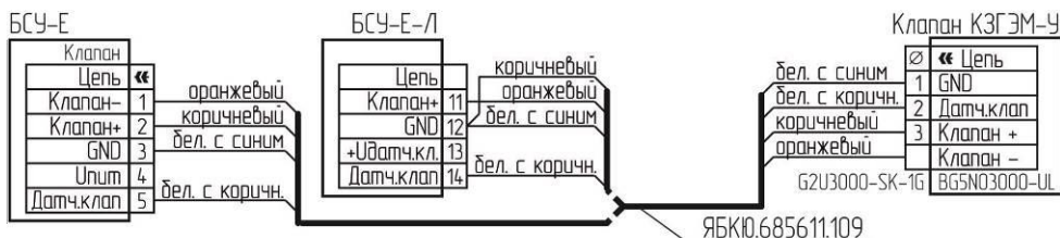
Рисунок Б.2 – Схема подключения клапана КЗГЭМ-У с разъемом BG5N03000-UL.
