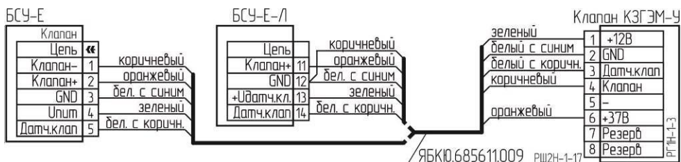
Рисунок Б.1 – Схема подключения клапана КЗГЭМ-У с разъемом P12H-1-3.
