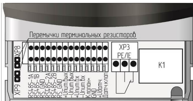
Рисунок А.3 – Расположение разъемов в клеммном отсеке БСУ-Е(Р)-Л1
