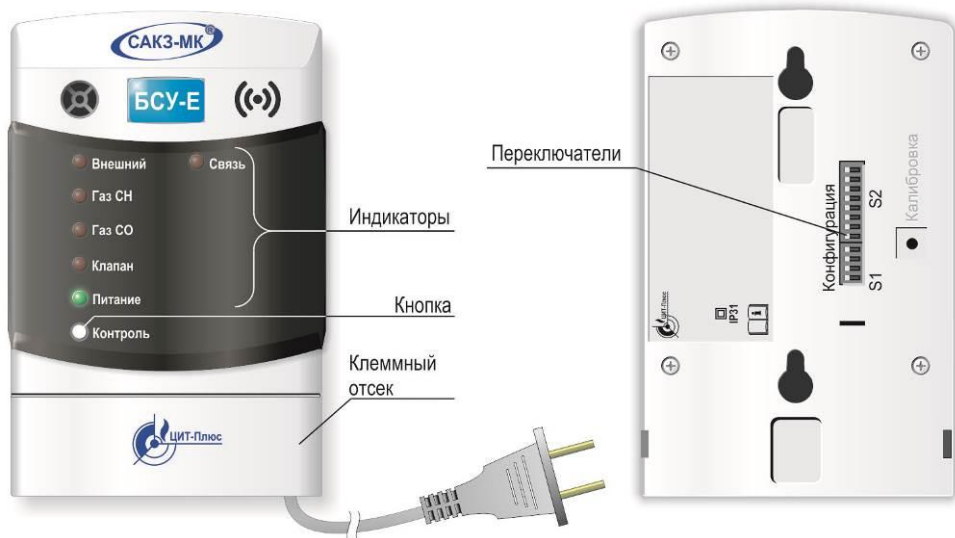
Рисунок 1 – Внешний вид блока (монтажная панель условно не показана).
