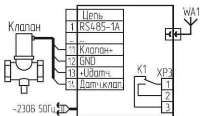
б) БСУ-ЕР-Л
