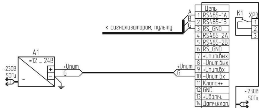
Рисунок 4 – Схема подключения БСУ-Е(Р)-Л к источнику вторичного электропитания
