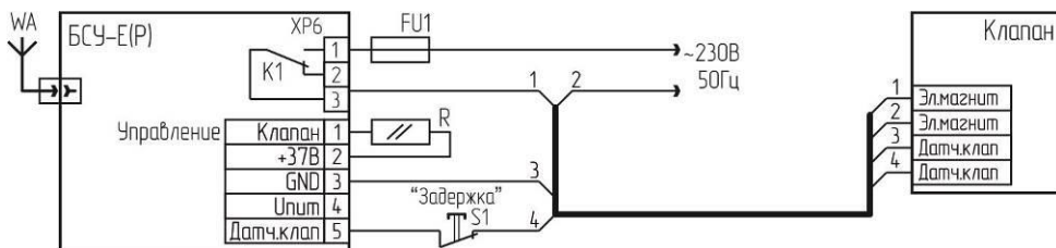
а) блок БСУ-Е(Р)
