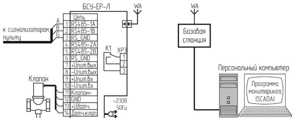
в) блок БСУ-E-P-Л в режиме LoRaWAN
