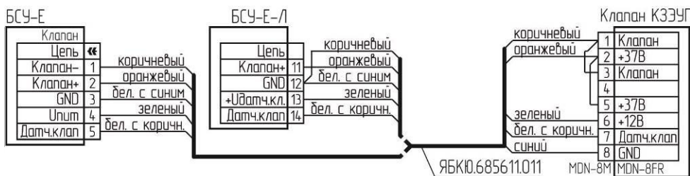
Рисунок Б.3 – Схема подключения клапана КЗЭУГ с разъемом MDN8FR.
