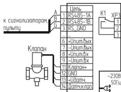
б) БСУ-Е-Л
